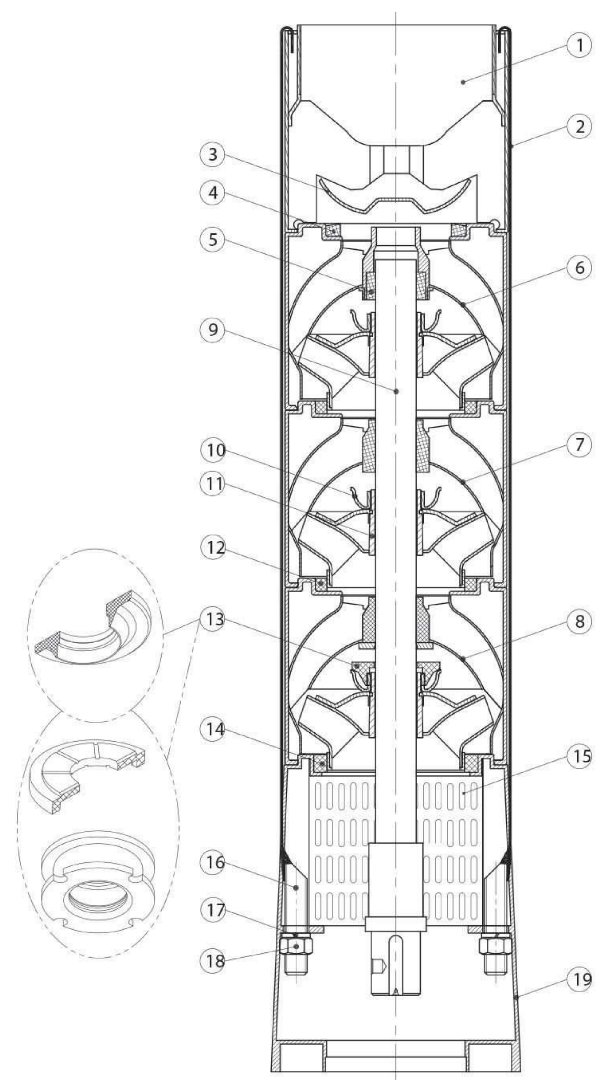
Pump 117-130-146-160
